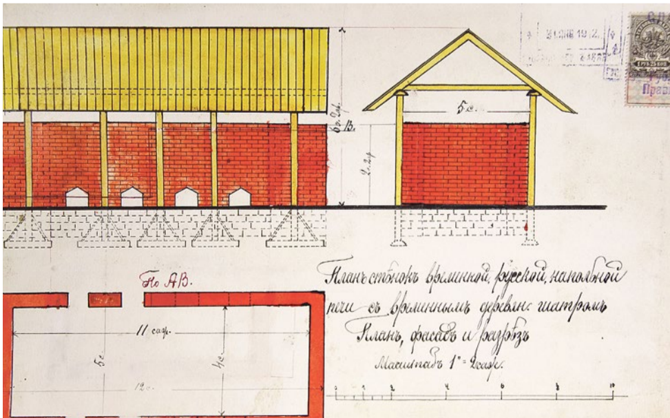
План временной русской напольной печи с временным деревянным шатром.
